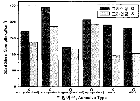
그림 5 접착면의 상태에 따른 전단접착강도
