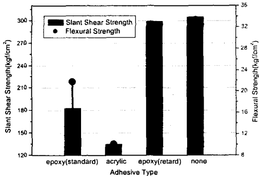
그림 3 접착제 종류에 따른 전단접착강도 및 휨접착강도
