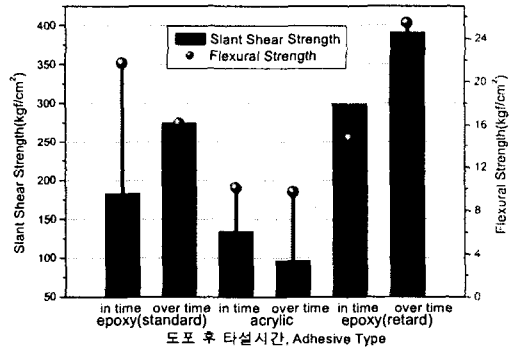
그림 4 콘크리트 타설시간에 따른 전단강도
