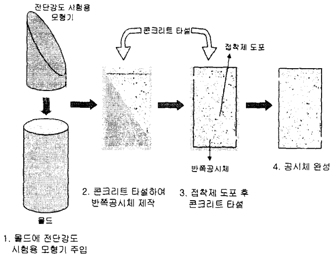
그림 1 전단강도 시험용 공시체 제작과정
