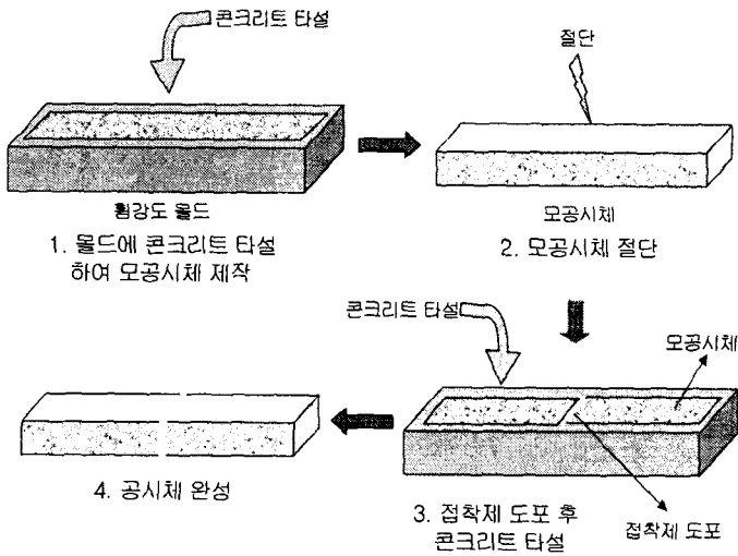
그림 2 휨강도 시험용 공시체 제작과정
