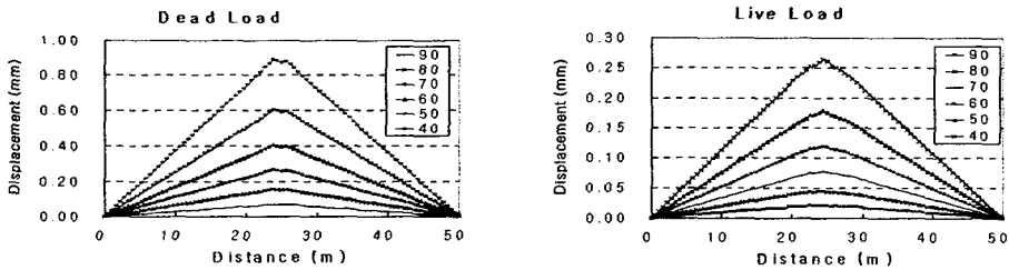
(a) 사하중에 의한 처짐값의 변화량 (b) 설계활하중(LS-22)에 의한 처짐값 변화량 그림 2 유효강성비(β)에 따른 처짐값 변화량
