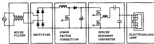
그림 5. SMPS형의 전극 전원장치의 구조 Fig. 5. SMPS type construction of power supply
