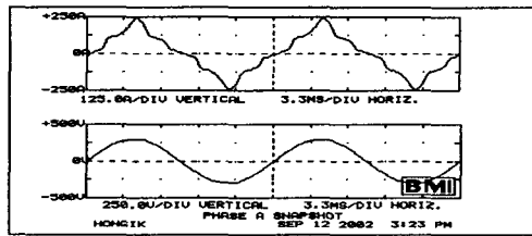
(a) A상 전류 및 전압파형
