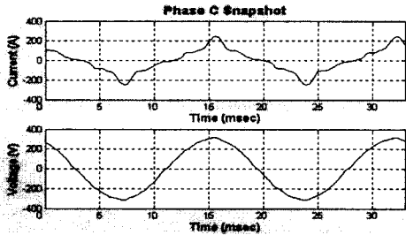
(a) C상 전류 및 전압파형
