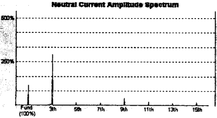
(b) 중성선 전류 스펙트럼
