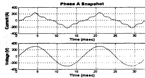
(a) A상 전류 및 전압파형
