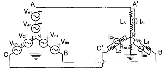
그림 9. 3상 등가 회로 Fig. 9. Three-Phase Equivalent Circuit
