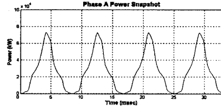
그림 14. A상 전력 파형 Fig. 14. Simulated Power Waveforms for Phase A
