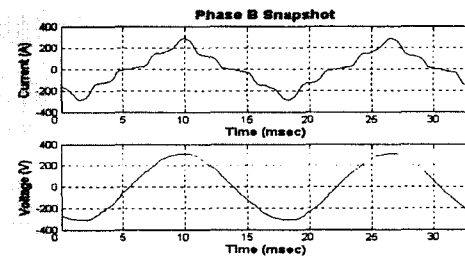
그림 10. A상 전류 및 전압 파형 Fig. 10. Simulated Current and Voltage Waveforms for Phase A
