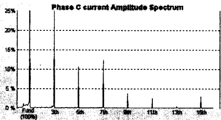
(b) C상 전류 스펙트럼
