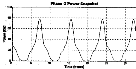
그림 16. C상 전력 파형 Fig. 16. Simulated Power Waveforms for Phase C
