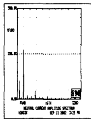
(b) 중성선 전류 스펙트럼
