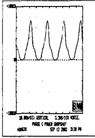
그림 8. C상 전력 파형 Fig. 8. Power Waveform for Phase C
