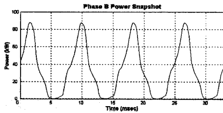
그림 15. B상 전력 파형 Fig. 15. Simulated Power Waveforms for Phase B
