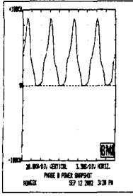
그림 7. B상 전력 파형 Fig. 7. Power Waveform for Phase B
