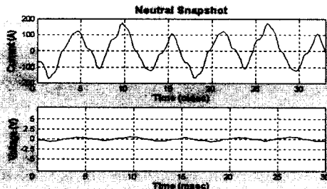
(a) 중성선 전류 및 전압파형
