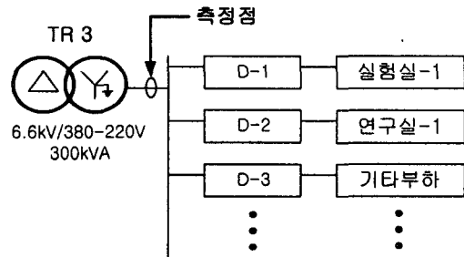
그림 1. 사례 연구 배전 시스템 Fig. 1. Single-line Diagram of the Distribution System Under Study
