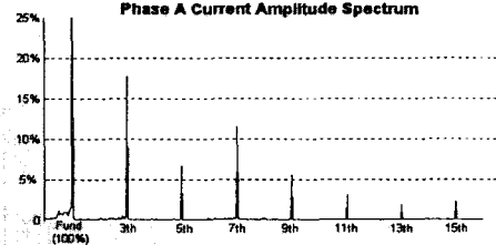
(b) A상 전류 스펙트럼
