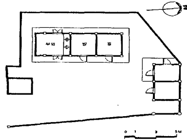
그림 3. 인곡리 공가
