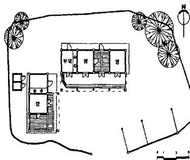
그림 4. 장곡리 박필녀씨가옥
