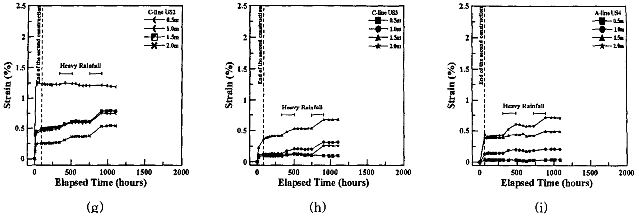
그림 17. 시간 경과에 따른 보강재의 유발 변형률
