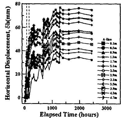
그림 14. 시간경과에 따른 수평변위 (A-Line)
