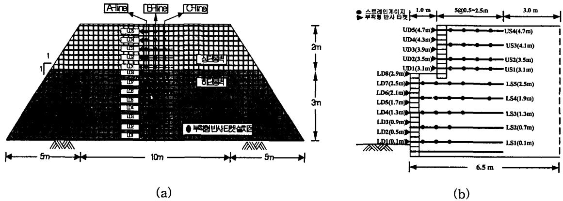
그림 9. 부착형 반사 타켓 설치 정면도 및 Strain gage 설치 전개도
