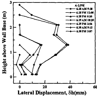
그림 10. 1단옹벽시공완료시 발생하는 수평변위
