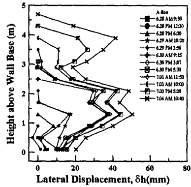
그림 11. 2단옹벽 시공완료시 발생하는 수평변위
