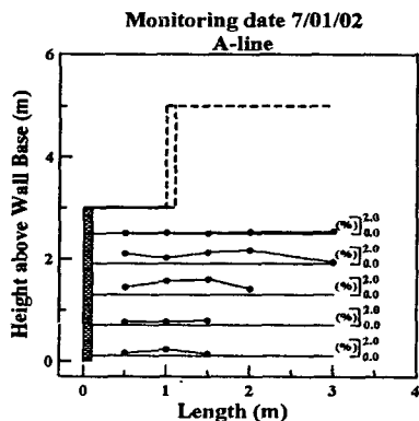
그림 15. 1단옹벽시공완료시 유발변위
