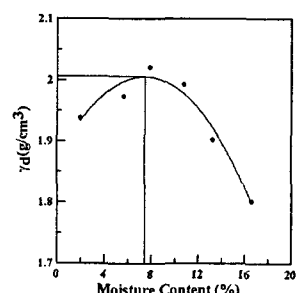
그림 6. 다짐시험결과
