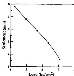
그림 5. 평판재하시험결과
