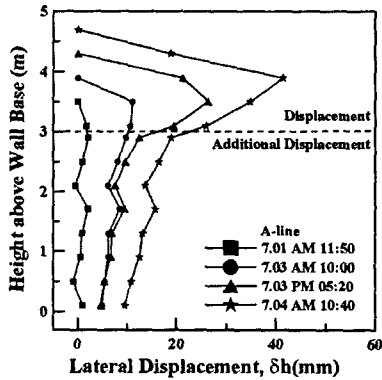
그림 12. 1단옹벽시공시 발생하는 추가변위
