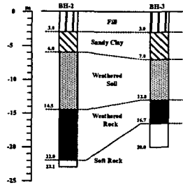
그림 2. 지반시험장의 주상도
