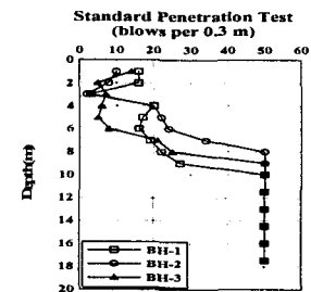
그림 3. 표준관입시험결과
