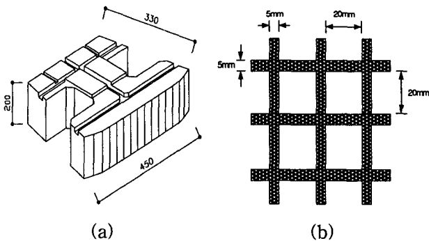
그림 7. RECO블록 및 지오그리드 제원
