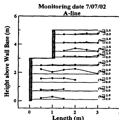
그림 16. 2단옹벽 시공완료시 유발변위
