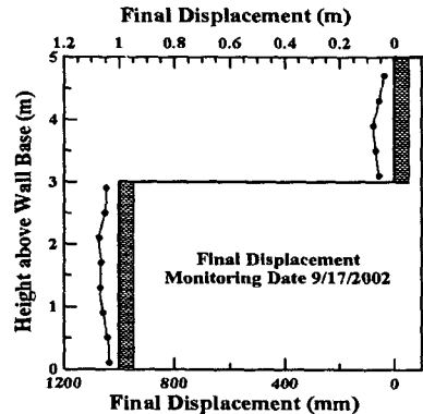
그림 13. 최종변위 (9/17/2002)
