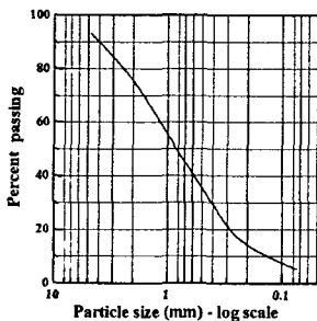
그림 4. 체분석시험결과
