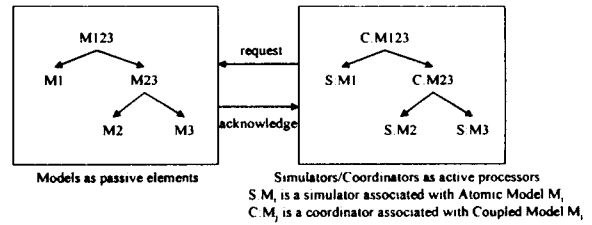
그림 1 추상화된 시뮬레이터의 구조
