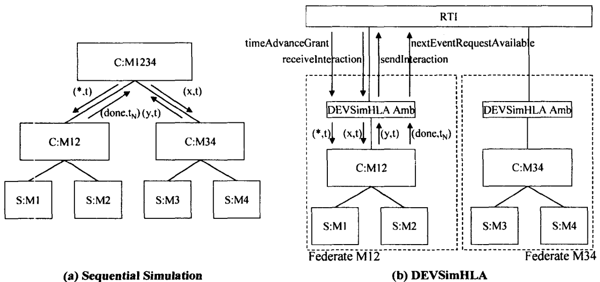
그림 3 DEVSimHLA의 구조와 메시지 변환
