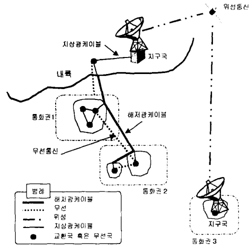
그림 1. 도서통신의 개념도
