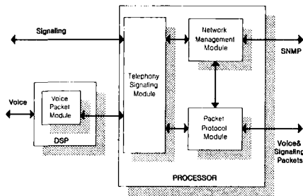
그림 1. 인터넷전화 기본 구조
