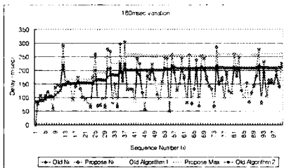
그림 8. 180msec 지연변동의 네트워크
