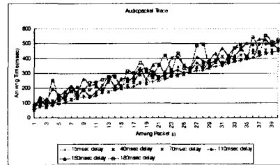
그림 4. 다양한 음성패킷트레이스
