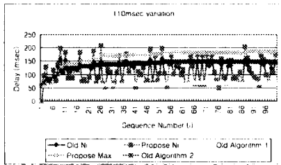
그림 7. 110msec 지연변동의 네트워크
