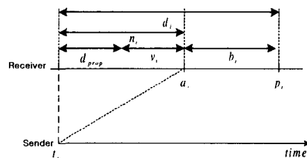
그림 3.패킷 i의 지연관계
