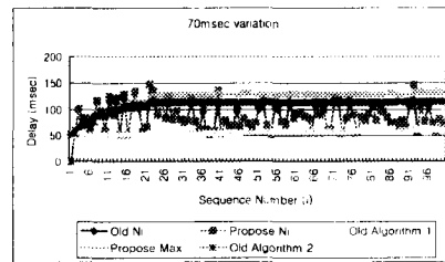
그림 6. 70msec지연변동의 네트워크
