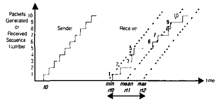
그림 2. 음성패킷의 생성과 재생
