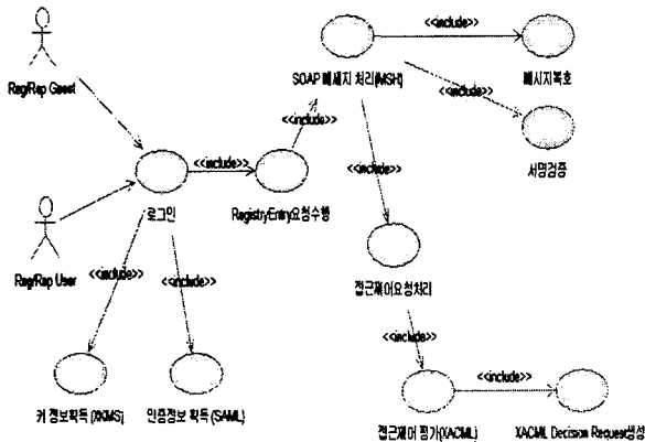
그림 1 Registry/Repository Usecase
