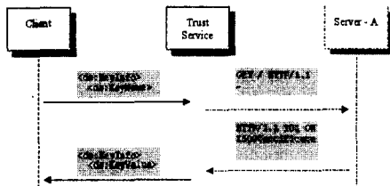
<그림 1> Tier1 Protocol의 구조
