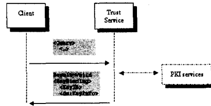
<그림 2> Tier 2의 키 검증 서비스 구조
