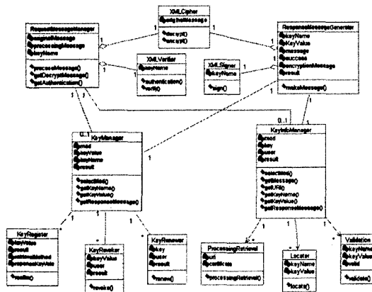
<그림 1> XKMS 웹 서비스 클래스 다이어그램
