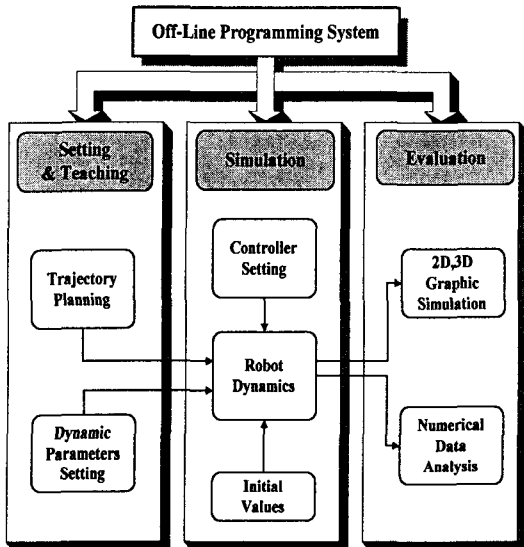
그림 2. 오프라인 프로그래밍 시스템의 구성
