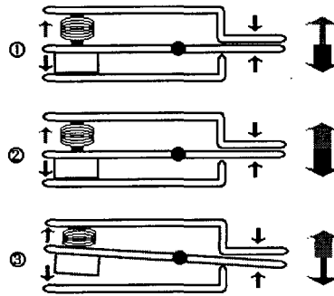
그림 2.7. 센서 동작시의 힘의 관계
