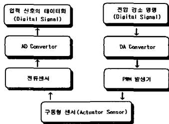
그림 2.8. 시스템 제어 블록도
