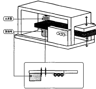
그림 2.5. 구동형 센서부
