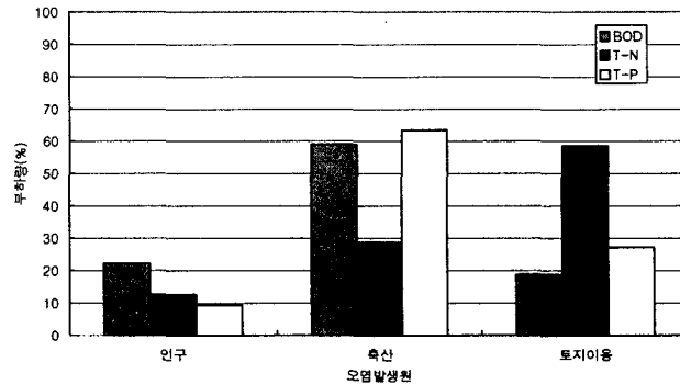
<그림 3> 오염 발생부하량 기여율
