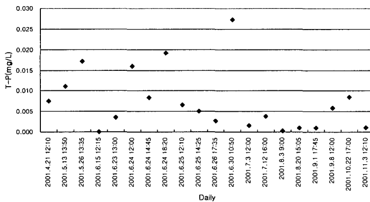
<그림 5(c)> 조사지점 시기별 T-P 농도 변화
