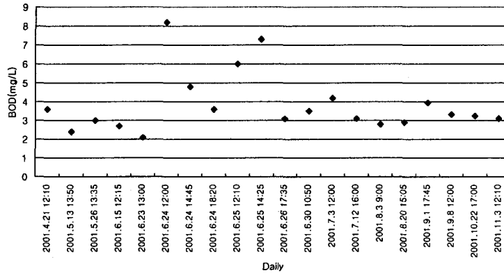
<그림 5(a)> 조사지점 시기별 BOD 농도 변화
