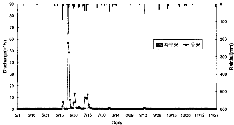
<그림 4> 조사유역의 일 유출량
