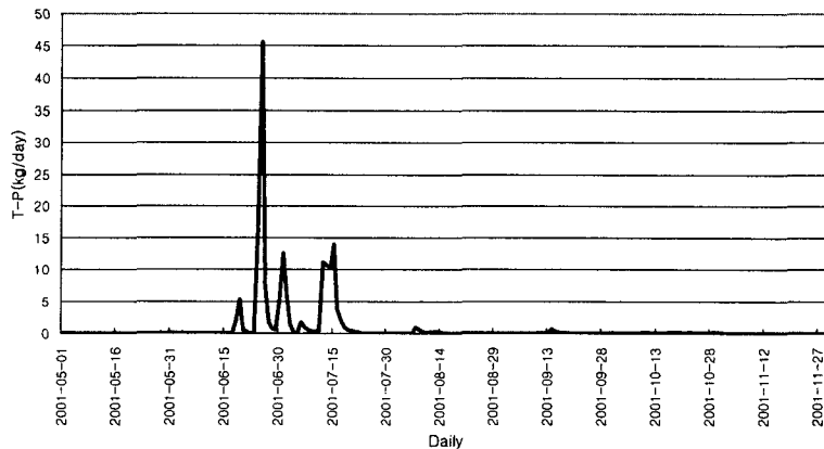
<그림 6(b)> 조사지점 T-P 일별부하량
