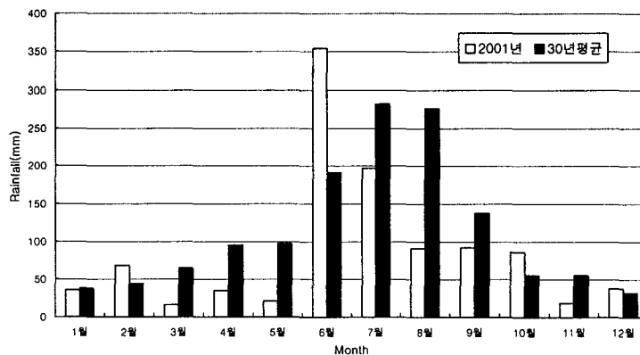
<그림 2> 평균 강수량과 2001년 강수량 비교
