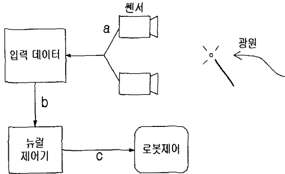
그림 5. 제어구조
