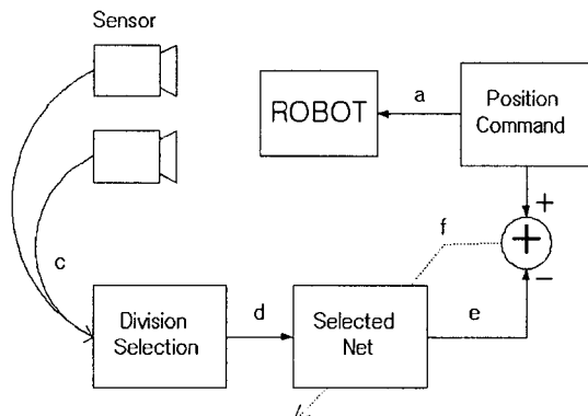
그림 4. 학습 구조
