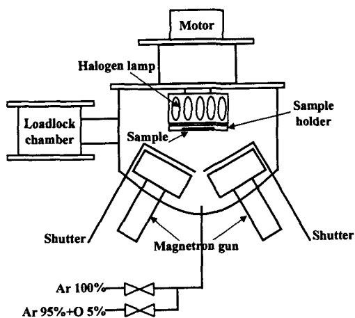
그림 1. rf 마그네트론 스퍼터링 시스템 개략도. Fig. 1. Schematic drawing of the rf magnetron sputtering system
