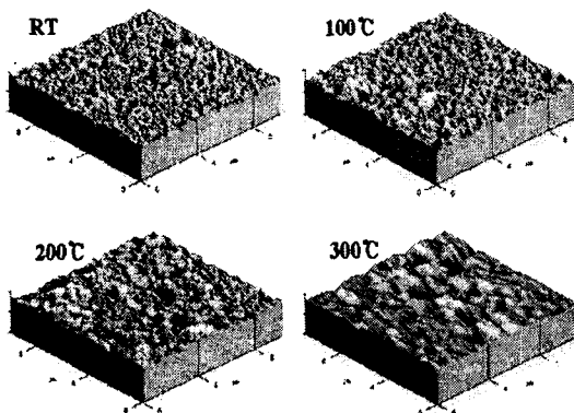
그림 7. 60초 에칭한 ZnO:Al 투명전도막의 표면 형태 Fig. 7. Surface morphology of the transparent ZnO:Al films as 60 second etching
