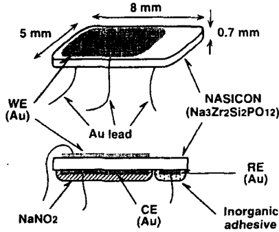
그림 1. 센서소자 Fig. 1. Solid electrolyte sensor configuration.
