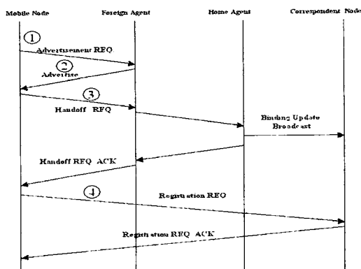
그림 1. Mobile IP의 동작
