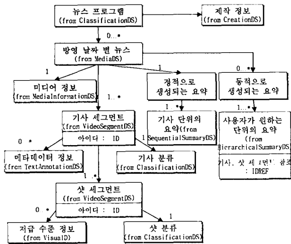
<그림 2> 뉴스 동영상 스키마 다이어그램
