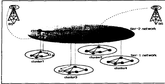
그림1. NSDR(New Secure Dynamic Routing Scheme)
