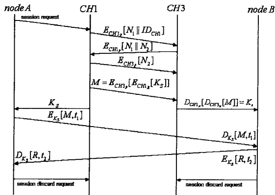
그림 2. 다른 클러스터내의 두 노드간 인증 알고리즘
