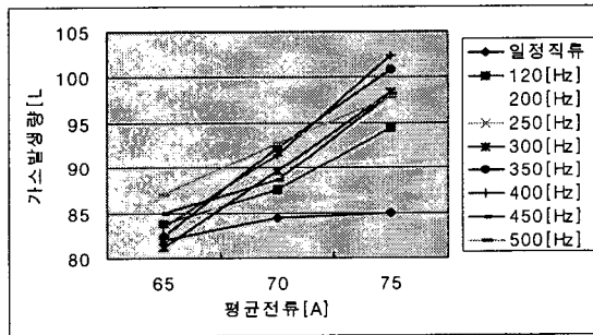
그림 9 포화영역에서의 가스발생량 Fig . 9 Gas generating- quantity at saturation region
