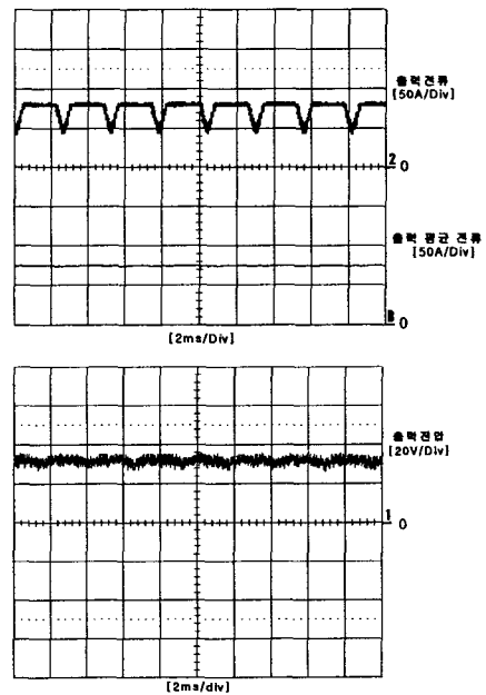
그림 7 주파수400[Hz]에서 부하전류[50A/div], 부하전압[20V/div] Fig . 7 Load current[50A/div], Load voltage[20V/div] at 400[Hz]
