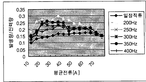
그림 10 각각의 평균전류에서의 입력전력당 가스발생량 Fig . 10 Gas generating- quantity per input power at each average current
