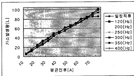
그림 8 일정직류 및 각 주파수에서의 가스발생량 Fig . 8 Gas generating- quantity at DC Current and each Frequency
