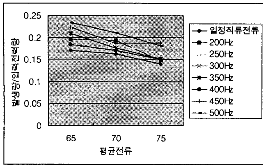
그림 11 평균전류 65[A], 70[A], 75[A]에서의 입력전력당 가스발생량
