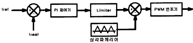
그림 2 제어블럭선도
