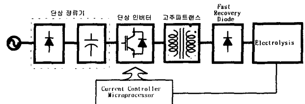
그림 1 인버터를 이용한 펄스전원의 블록선도
