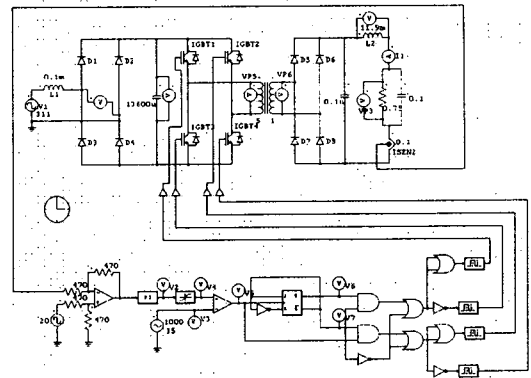
그림 4 시뮬레이션 회로도
