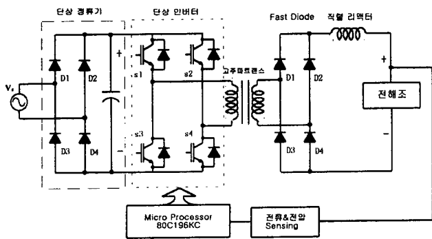
그림 3 전기분해용 펄스전원
