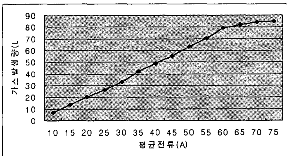
그림 6 일정 직류전류 인가시 가스발생량 Fig . 6 Quantity of gas generation at DC current
