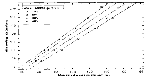
그림 8 와이어 용융속도와 극성비의관계
