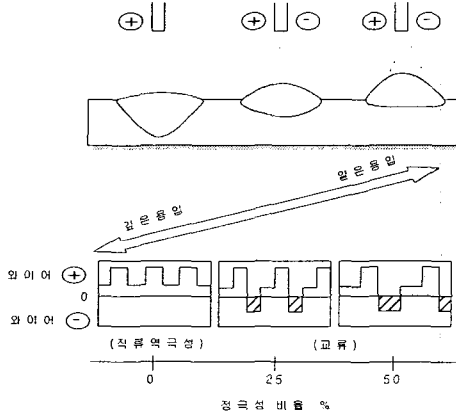
그림3 극성비율과 용입 형상과의 관계
