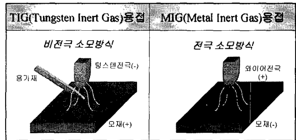
그림1 TIG용접과 MIG용접의 비교
