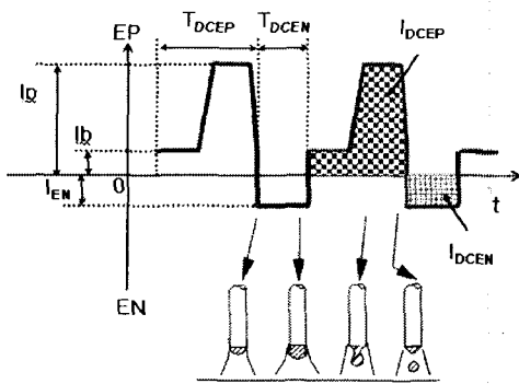
그림2 펄스MIG 용접의 용접알고리즘
