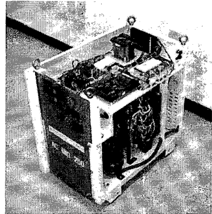
그림 12 제작된 펄스 MIG용접장치 시작품
