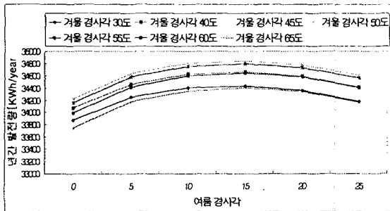
그림 5 계절별 조절 방식에 따른 연간 발전량
