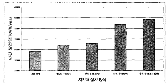
그림 7 지지대 설치방식에 따른 연간 발전량
