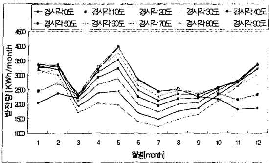
그림 4 경사각의 변화에 따른 월별 발전량
