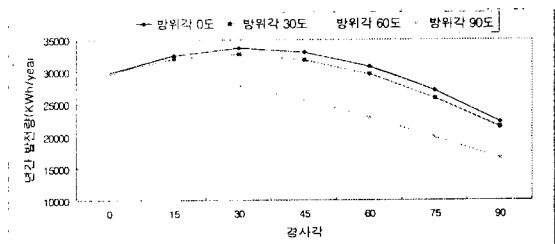
그림 3 경사각과 방위각에 따른 년간 발전량
