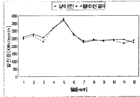
그림 2 시뮬레이션에 의한 PV시스템의 월별 성능결과
