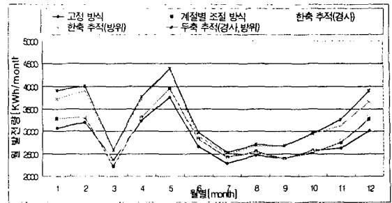
그림 6 지지대의 설치 방식에 따른 월별 발전량
