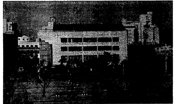
그림 1 30kW급 계통연계형 태양광 발전시스템
