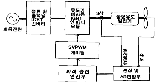
그림 2 시스템 구성도
