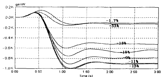
그림 9 일정속도-슬립변동에 의한 출력파형 Fig. 9 Slip - Output Power wave form
