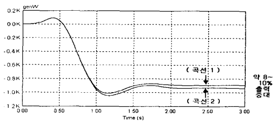
그림 8 SPWM-SVPWM 출력비교 Fig. 8 Compare the Output Power between SPWM and SVPWM
