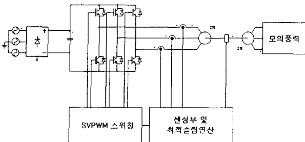
그림 6 최대출력 제어시스템 시뮬레이션 구성도 Fig. 6 Simulation block for optical power control system
