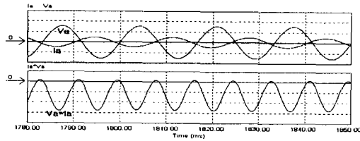
그림 5 시뮬레이션 전압 전류 및 순시전력 파형 Fig. 5 Voltage, current, power wave by simulation
