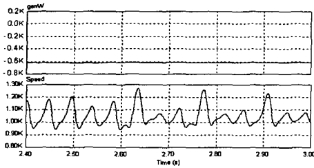
그림 10 속도변동시 출력파형 Fig. 10 Output Power at variable speed
