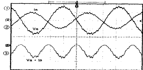
그림 3 농형 유도 발전기의 출력 파형
