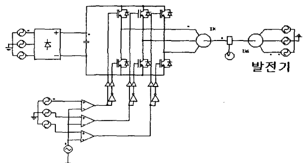
-그림 4 농형 유도발전기 시뮬레이션 구성도
