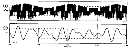
그림 7 발전기 출력단 전압전류 파형 Fig. 7 Voltage and current wave in generator
