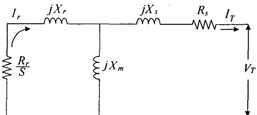
그림 1 유도발전기 등가모델
