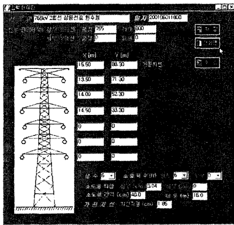
그림 4. TLCALC 2001 입력데이터 화면 예시 (2회선)
