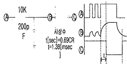
[그림5] 엔코드
