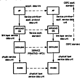
[그림 3] 계층별 통신 프로토콜 [Fig.3] Communication protocol by layer
