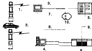
[그림 1] 정산 시스템의 구조 [Fig.1] A structure of ETC system
