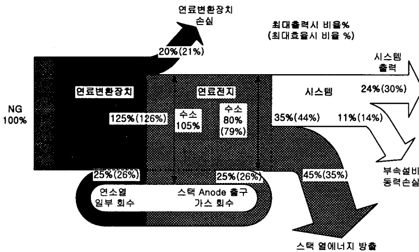
그림 6. 고분자 연료전지 시스템의 효율
