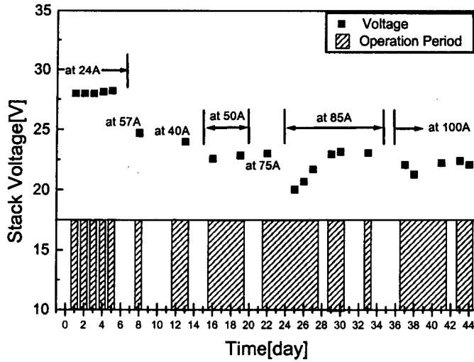
그림 5. 고분자 연료전지 스택의 장기 운전 특성
