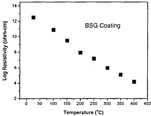
그림 5. 온도변화에 따른 소다붕규산염 유리의 전기비저항.
