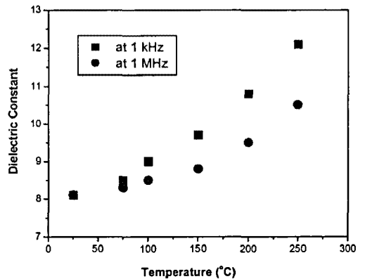
그림 4. 온도변화에 따른 소다붕규산염 유리의 유전상수.
