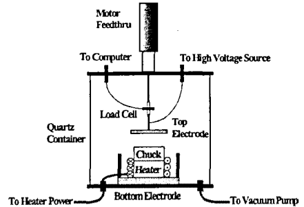
그림 1. 고착압력 측정장치의 도식도
