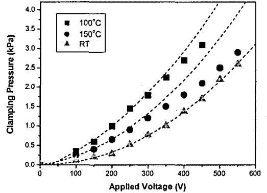
그림 3. 온도에 변화에 따른 소다붕규산염 유리/스테인레스스틸 ESC의 고착압력. Fig. 3. Clamping pressure of soda borosilicate glass/stainless steel ESC at various temperatures.
