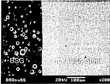
그림 2. 소다붕규산염 유리/스테인레스스틸 계면에서의 주사전자현미경 미세조직. Fig. 2. SEM micrographs at soda borosilicate glass/stainless steel interfaces.
