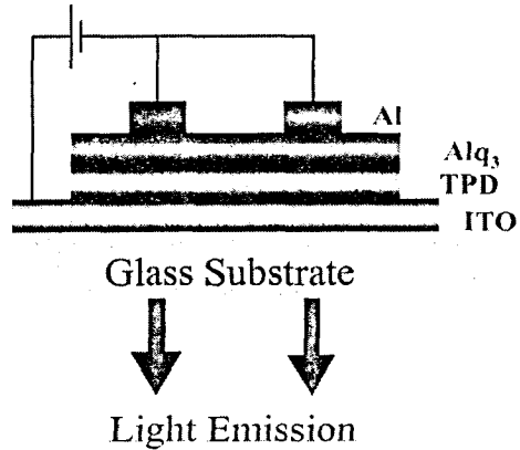
그림 2. 유기 발광 소자의 구조.
