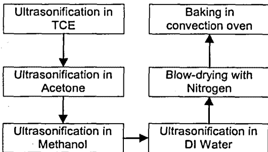
그림 1. ITO coated glass 세정공정 Fig. 1. Cleaning process of ITO coated glass
