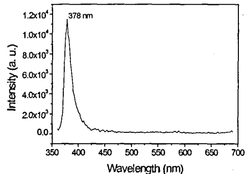
그림 2. ZnO 박막의 PL spectra
