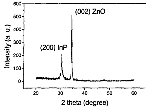
그림 1. ZnO 박막의 XRD pattern
