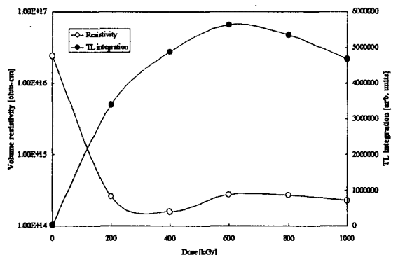
그림 3. 방사선 조사에 따른 체적저항율 및 집적 열발광량 ( 50\sim 250^{\circ}\text{C} )
