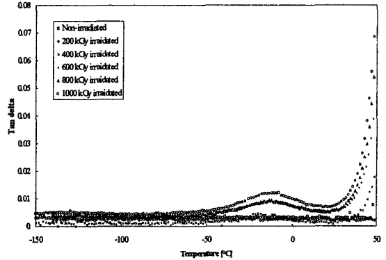
그림 2. \tan \delta 의 조사선량 및 온도 의존성
