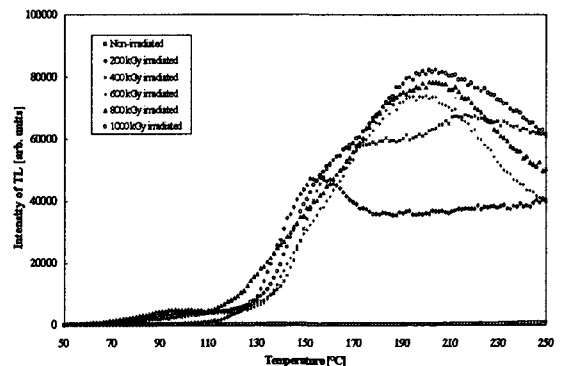
그림 1. 방사선 조사에 따른 열발광 스펙트럼
