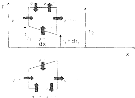
Fig. 5 에너지평형도
