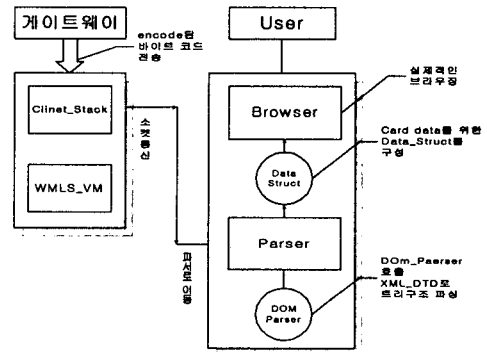
그림 1 WAP Emulator의 전체 구조도
