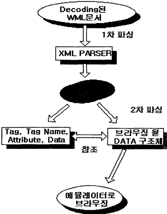
그림 2 WML 문서의 내부 처리 과정
