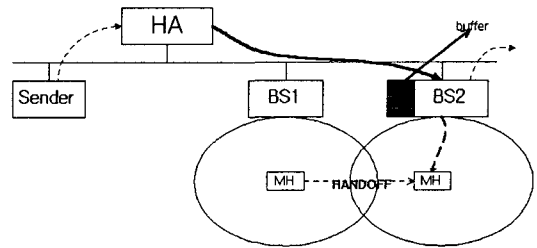
(그림 4) 핸드오프 완료후의 패킷 전달 경로
