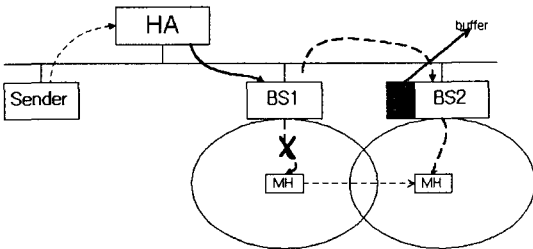
(그림 3) 핸드오프 실행 중의 패킷 전달 경로
