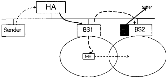
(그림 2) 핸드오프가 발생하기 전의 패킷 전달 경로
