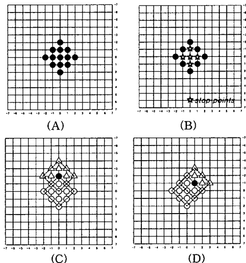
그림 1 . Modified Diamond Search Algorithm
