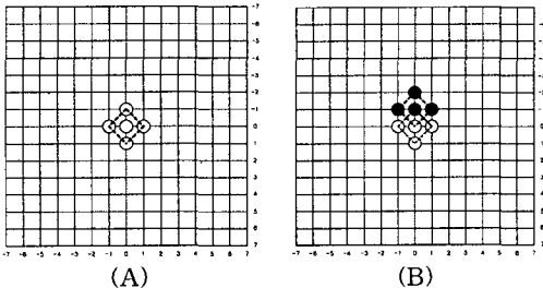
그림 3 Small Diamond Search Algorithm
