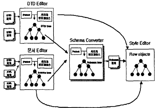
[그림 2] 시스템 구성도
