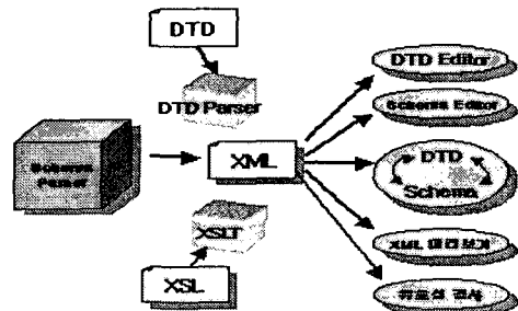
[그림 3] 스키마 Converter의 구조도
