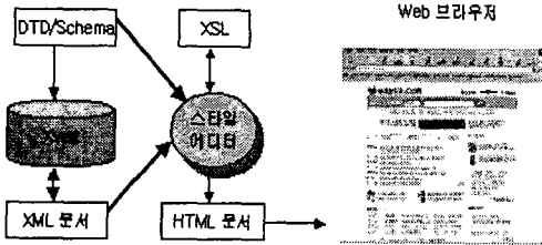
[그림 4] 스타일 에디터의 구조도
