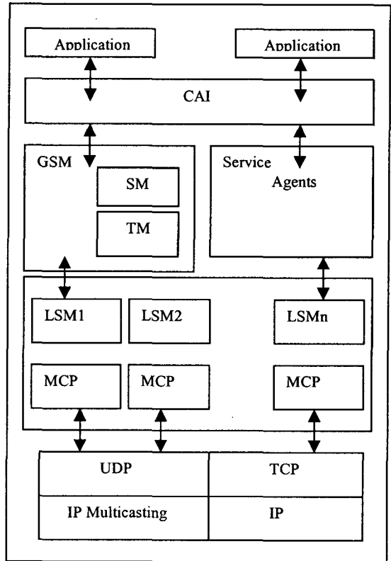
(그림 1) 객체지향 멀티미디어 협력 작업 프레임워크
