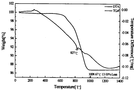
그림 2. BZCT 분말의 DT/TGA
