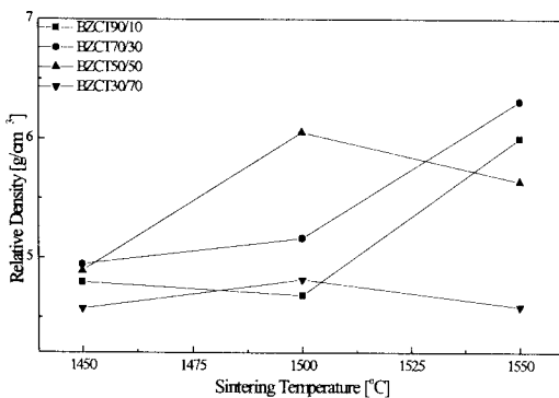
그림 6. 소결온도와 조성에 따른 BZCT 시편의 밀도
