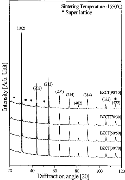
그림 5. 조성에 따른 BZCT 시편의 X-선 회절모양
