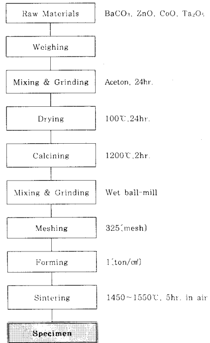
그림 1. BZCT 세라믹스의 제조공정
