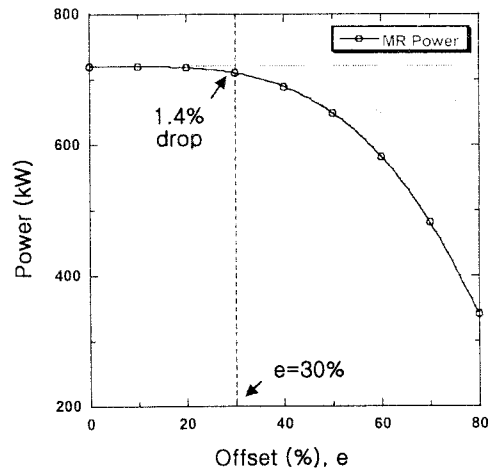
그림 4. 블레이드의 휨셋에 의한 파워곡선
