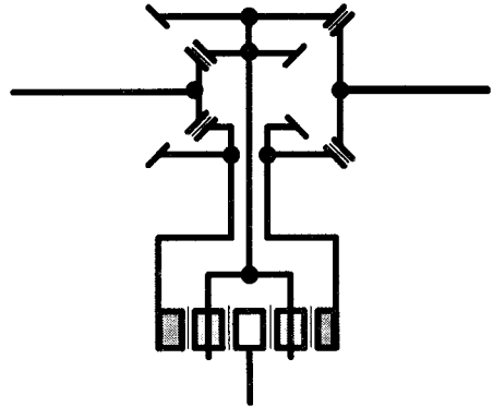
(그림 3) 특수 베벨-유성 기어 개략도
