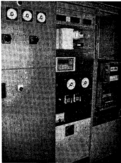
그림 2. 계측설비 및 제어설비
