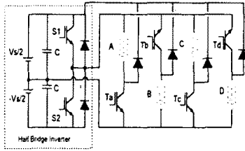
그림 2. 하프 브리지 인버터형 SRM 컨버터 토폴로지
