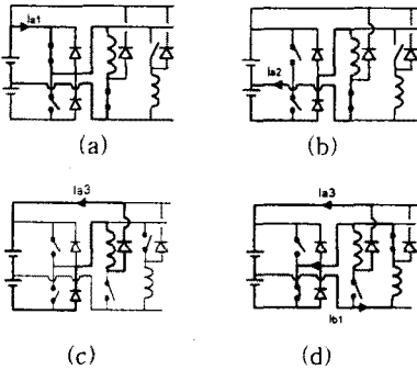
그림3. 하프브리지 인버터형 SRM 컨버터의 4가지 동작 모드(a) 모드 I (b) 모드 II (c) 모드 III (d) 모드 IV
