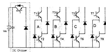
그림 1. 직류초퍼가 삽입된 비대칭 브리지 SRM 컨버터
