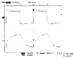
그림 6. 위상방식시 인버터에서 나타나는 출력전압과 출력전류
