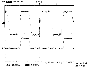
그림 5. 초핑제어시 인버터측의 출력 전류와 컨버터측의 상전류
