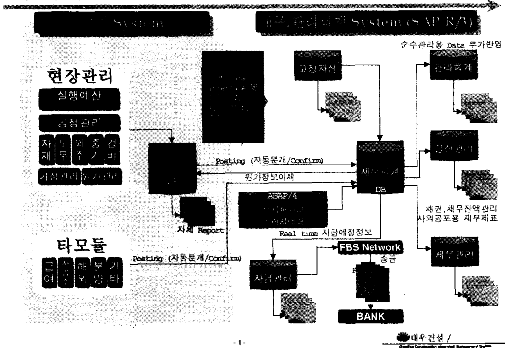
<그림 2> DW-CIMS의 개요도
