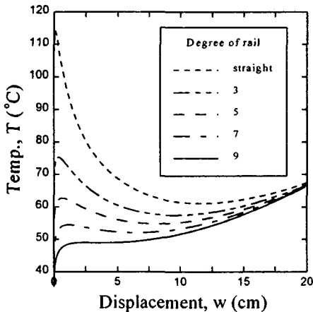
그림 5. 궤도곡률에 따른 좌굴온도 곡선
