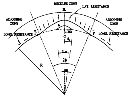
그림 2. 곡선 CWR 궤도의 좌굴전과 좌굴후의 형상
