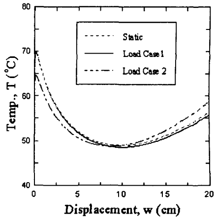
그림 13. 정적과 동적좌굴 비교
