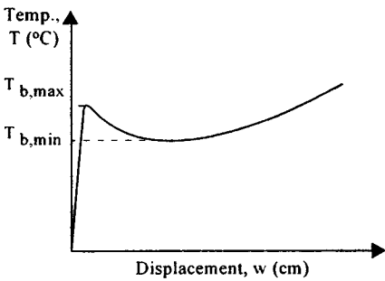
그림 1. 좌굴온도 곡선
