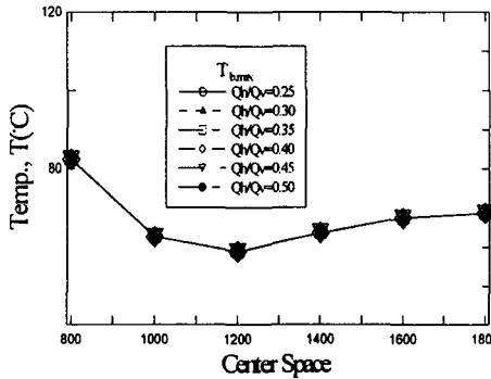
그림 11. 상부좌굴온도에 미치는 Q_H/Q_V 비의 영향
