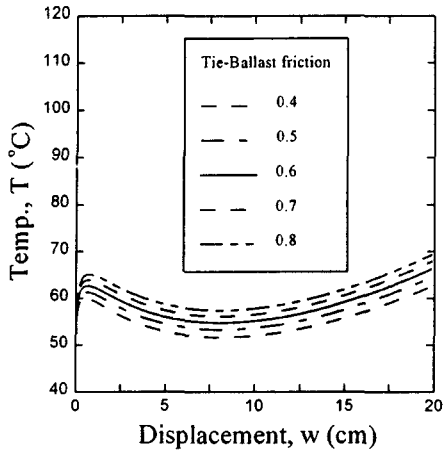
그림 9. 침목 바닥고 도상 마찰계수에 따른 좌굴온도 곡선
