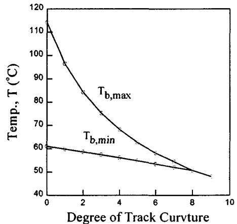
그림 6. 궤도 곡률의 영향
