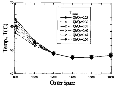
그림 12. 하부좌굴온도에 미치는 Q_H/Q_V 비의 영향
