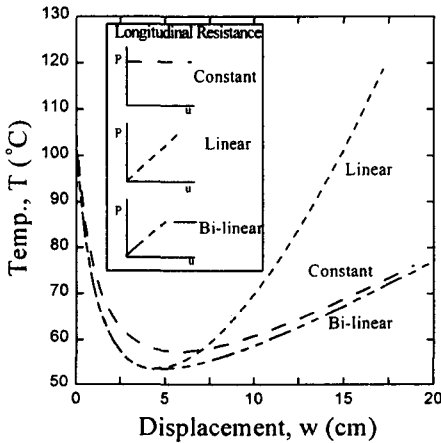
그림 7. 종방향저항 특성에 따른 좌굴온도
