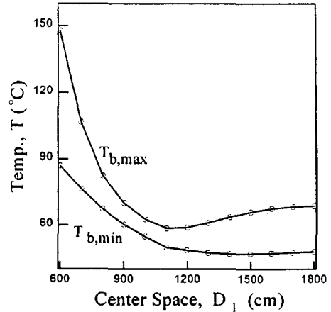
그림 10. 대차 중심간 거리변화에 따른 좌굴온도
