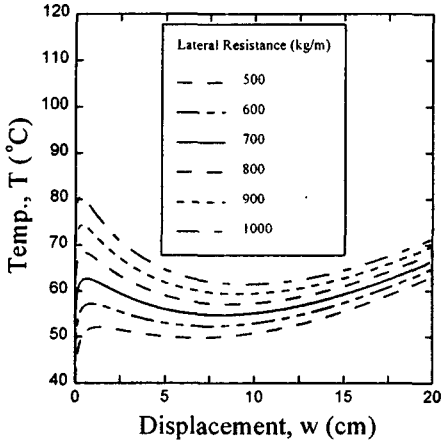
그림 3. 횡방향 저항에 따른 좌굴온도 곡선
