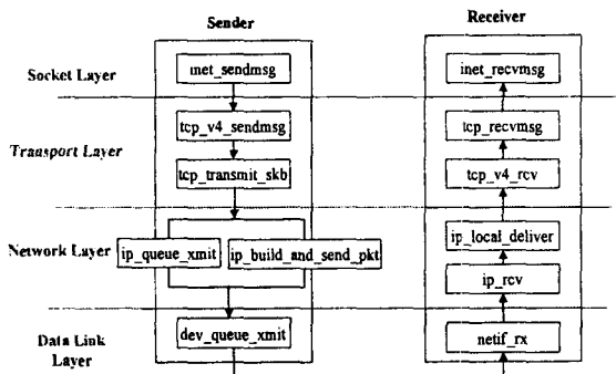
그림 4: 리눅스의 Normal TCP/IP 흐름도
