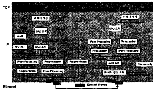
그림 5: IP 계층에 통합된 IPsec 처리 흐름도
