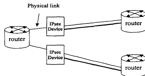
그림 3: BITW(Bump-in-the-Wire)
