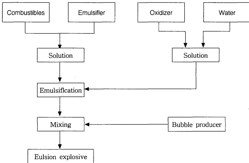
Fig. 1 에멀션 폭약의 제조공정도
