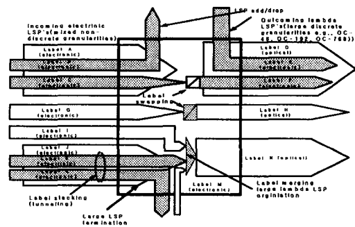
(그림3-1)전자적인 LSR기능과 혼합된 에지 광 LSR 기능
