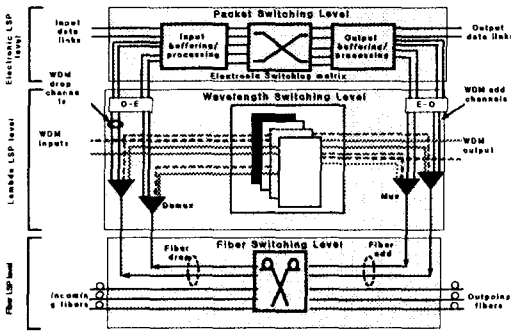
(그림3-2) 여러 단계의 레이블 스택을 갖는 FWP 교환 노드 구조
