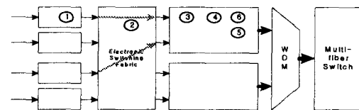
(a)전기적인 입력 패킷 처리 과정
