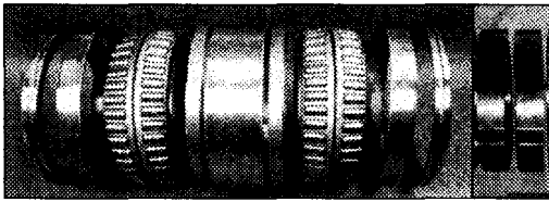
그림1. 압연기 베어링의 구조
