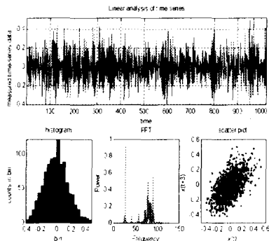
그림 2. 베어링 진동신호의 시계열과 히스토그램, FFT, 재구성한 어트랙터
