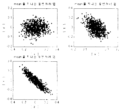
그림 6. 진동 신호의 포엔카레 단면
