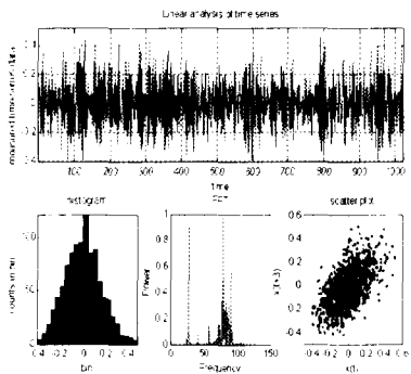
그림 3. 베어링 진동신호의 시계열과 히스토그램, FFT, 재구성한 어트랙터
