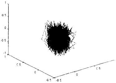
그림4. 3차원으로 재구성한 진동신호의 어트랙터
