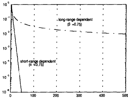
그림 97. 장기 의존성과 단기간 의존성의 비교
