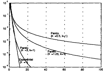
그림 98. Pareto 및 지수 확률 밀도 함수
