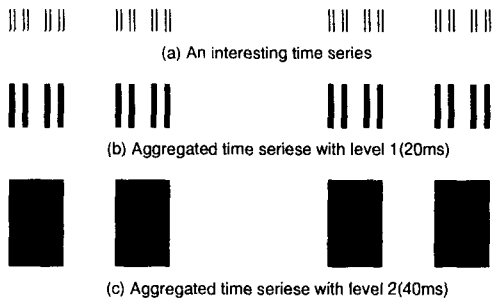
그림 96. Self-similar 시계열(time series).
