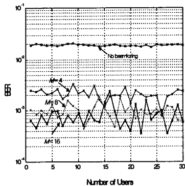
그림 6. Steering 빔포밍의 성능 시뮬레이션 결과
