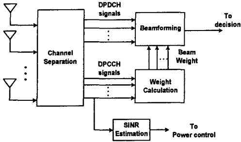
그림 1. WCDMA 시스템에 대한 기저대역 빔포밍 적용 구조도
