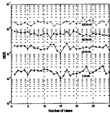
그림 5. 심볼단위 LMS 빔포밍의 성능 시뮬레이션 결과. M=4
