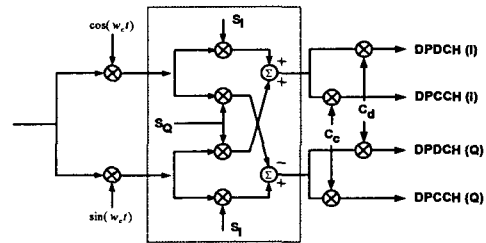
그림 2. WCDMA 시스템에서의 채널 복조 구조
